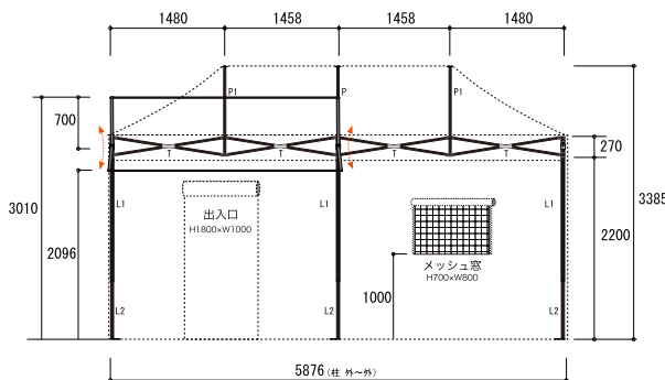
軸組図 (1)
