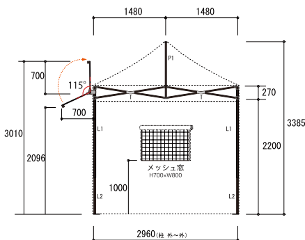
軸組図 (2)
